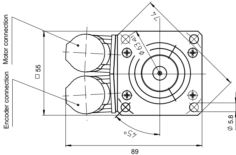
Motor type SR-A0
